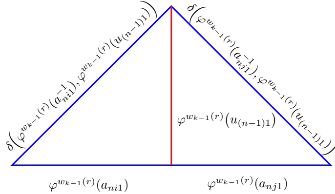
FIGURE 5.3. The van Kampen diagram \Delta_{ij}^n(w_k(r)) .
